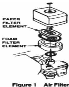
Рисунок 1. Воздушный фильтр
